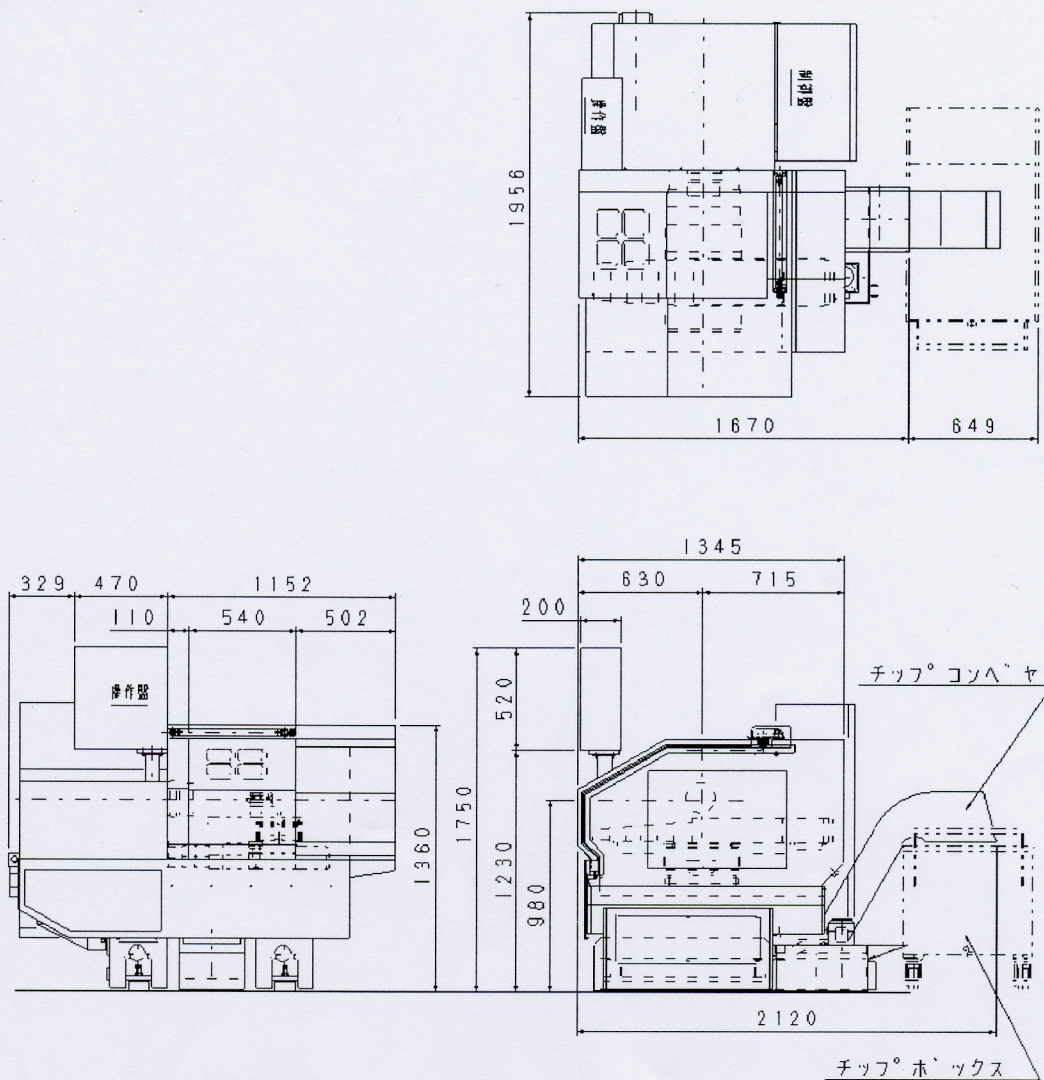
機械概略寸法 Floor space
