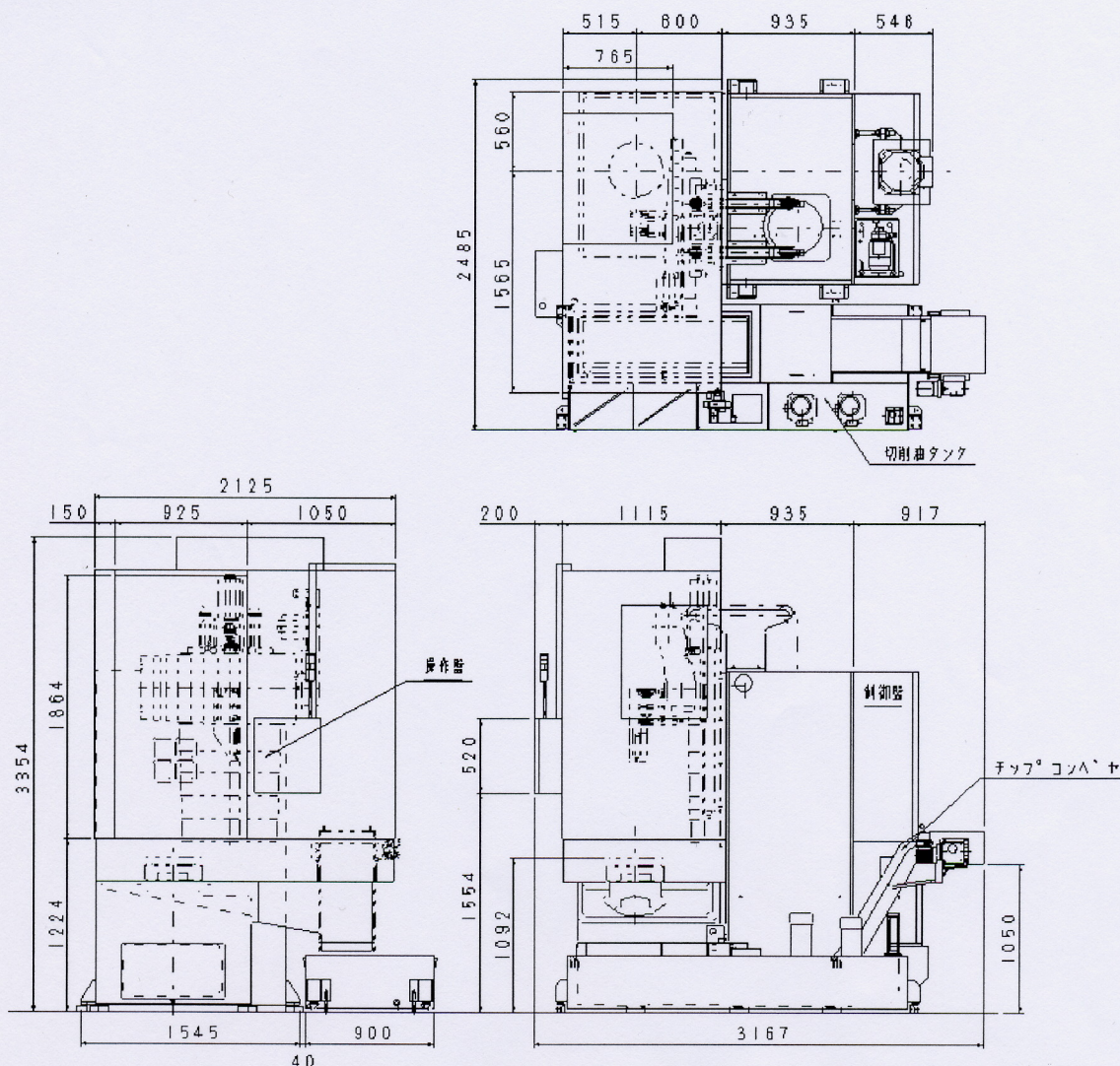
機械概略寸法 Floor space
